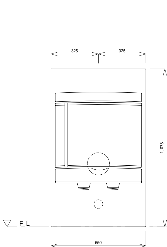
立面図
