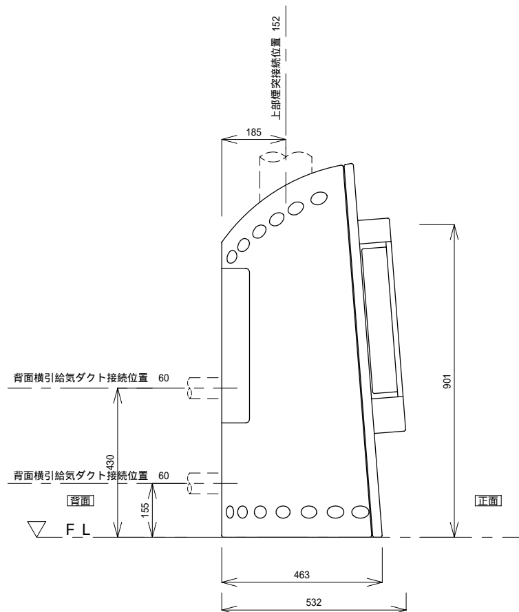
側面図
