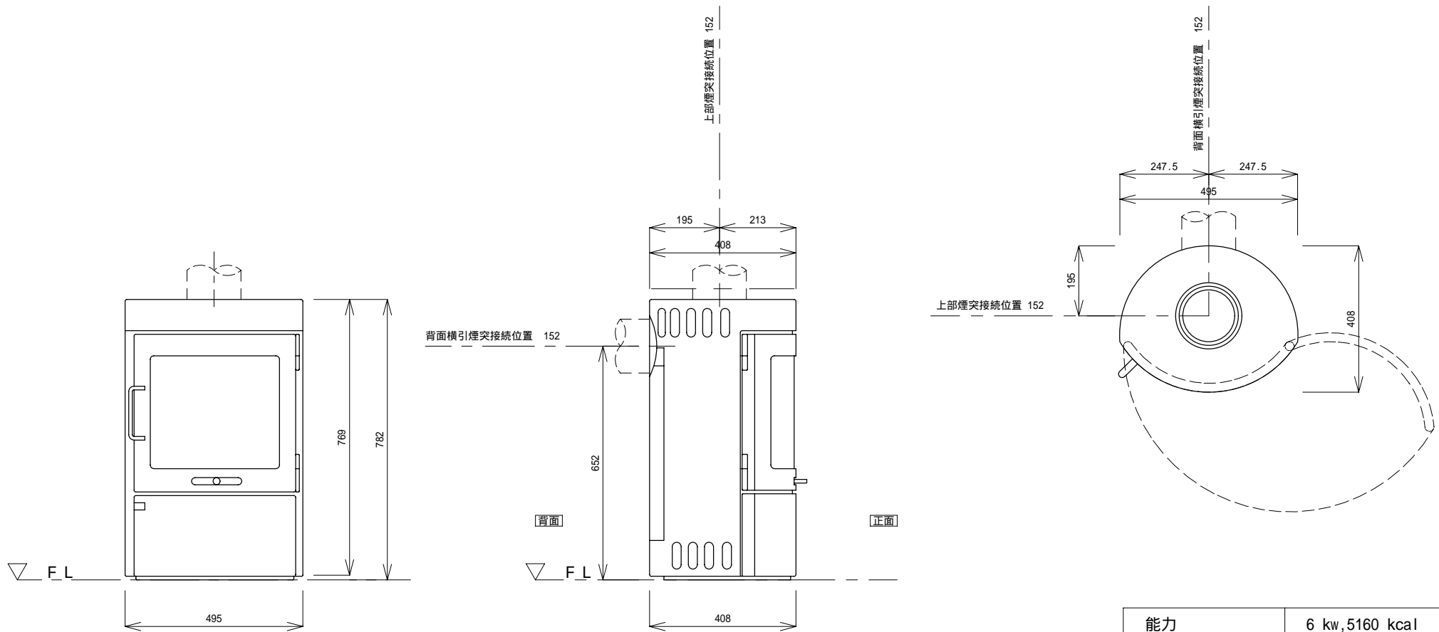
立面図
